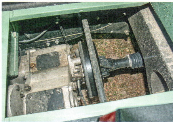
Ezt látjuk, ha kivesszük a középső ülés lapját: a kardán és alatta az út
